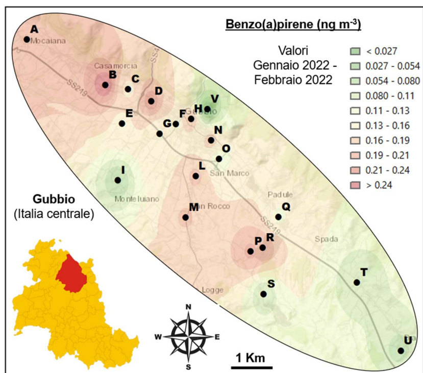
Figura 46. Mappatura spaziale della concentrazione del benzo(a)pirene nel \text{PM}_{10} durante il periodo di misura gennaio-febbraio 2022 nell'intera area di Gubbio.
